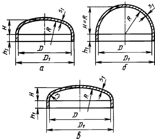
Выпуклые днища
