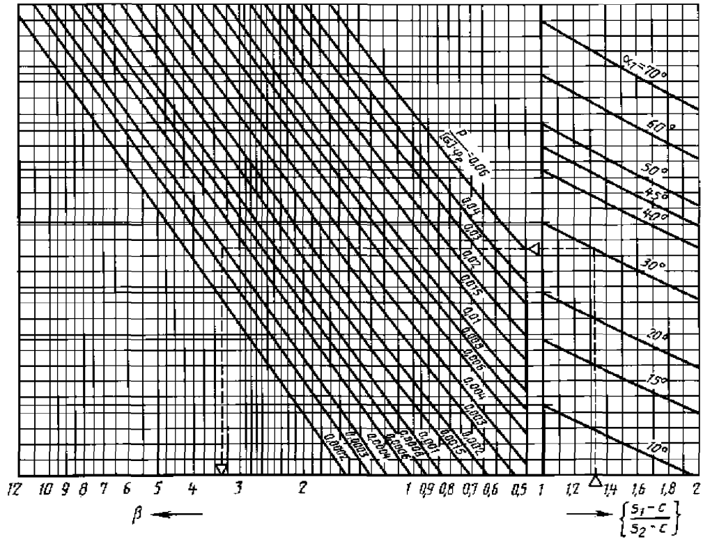
Диаграмма для определения коэффициента \beta при расчете толщин стенок переходов обечаек
